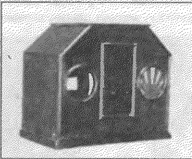
Телевізор Дж.-Л. Берда «Model «В»». Великобританія, 1928 р.
