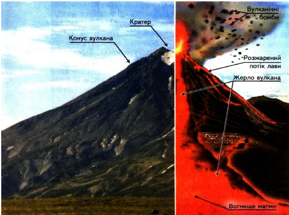
мал. 30. Будова вулкана
