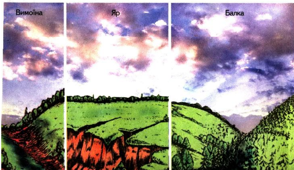
мал. 35. Робота текучих вод
