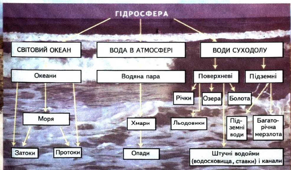
Мал. 73. Складові гідросфери
