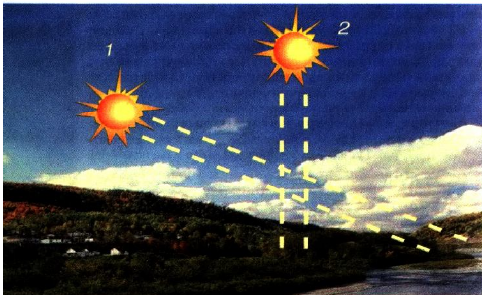
Мал. 56. Залежність ступеня нагрівання земної поверхні від кута падіння сонячних променів: 1 – кут падіння невеликий, а площа обігрівання значна, тому температура нагрівання невисока; 2 – кут падіння прямий, площа обігрівання невелика, тож температура нагрівання висока
