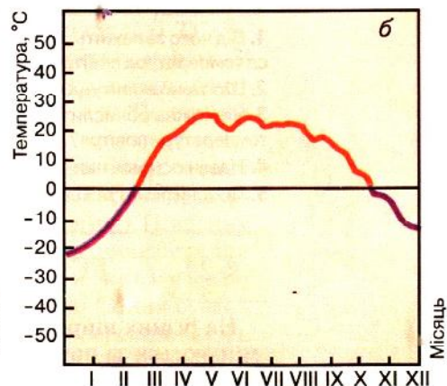
Мал. 57. Графіки ходу температур: а – добовий; б – річний
