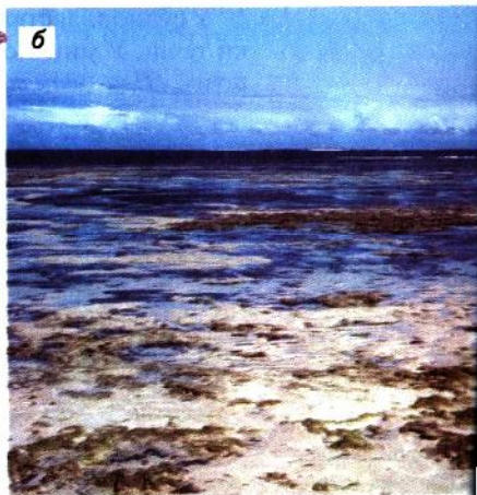
Мал. 81. Узбережжя моря під час: а — припливу; б — відпливу
