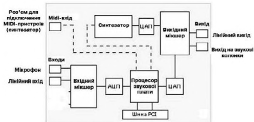
Рис. 2.18. Структура звукової плати
