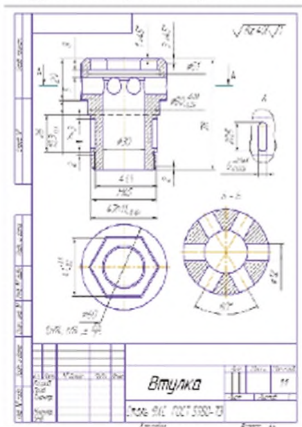
Рис. 5.3. Креслення, виконане в системі автоматизованого проектування
