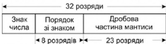
Рис. 1.1. 32-розрядне подання числа з плаваючою комою
