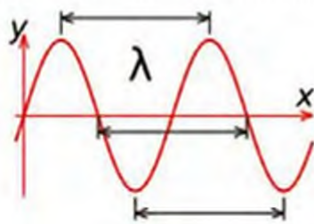
Рис. 2.12. Характеристики хвилі
