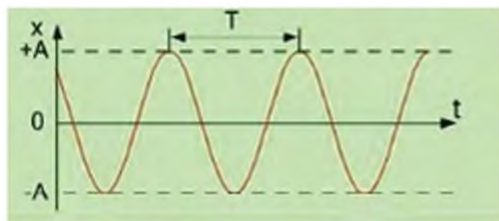
Рис. 2.11. Синусоїдальне коливання
