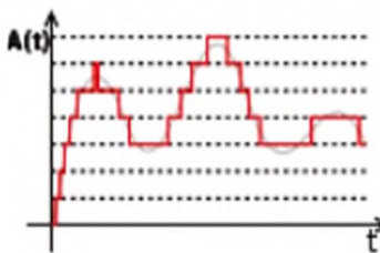
Рис. 2.15. Квантування сигналу
