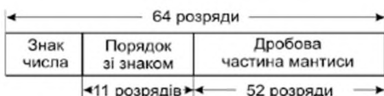
Рис. 1.2. 64-розрядне подання числа з плаваючою комою
