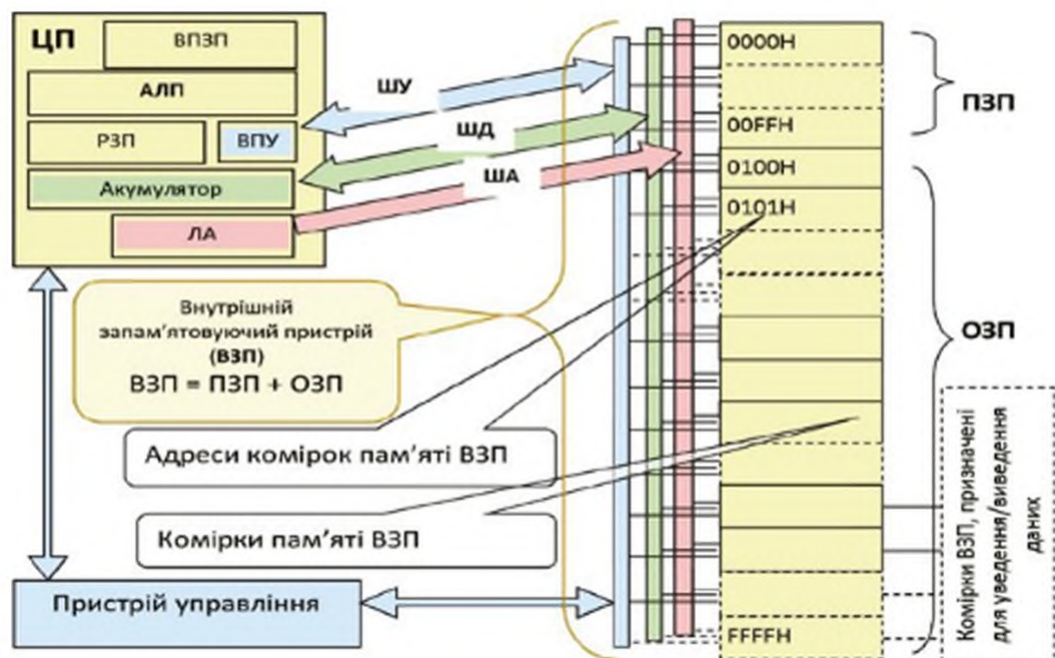
Рис. 3.1. Спрощена схема комп'ютера
