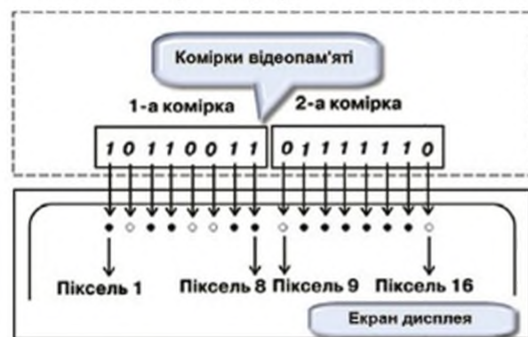
Рис. 2.6. Схема подання зображення у відеопам'яті
