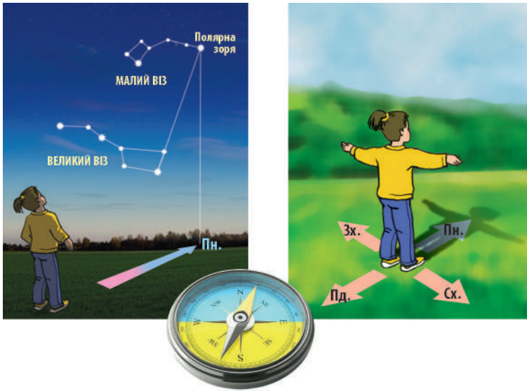
Способи визначення сторін світу
