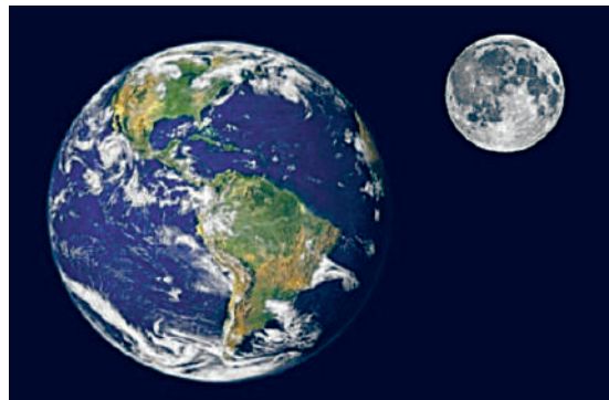
Система Земля — Місяць
