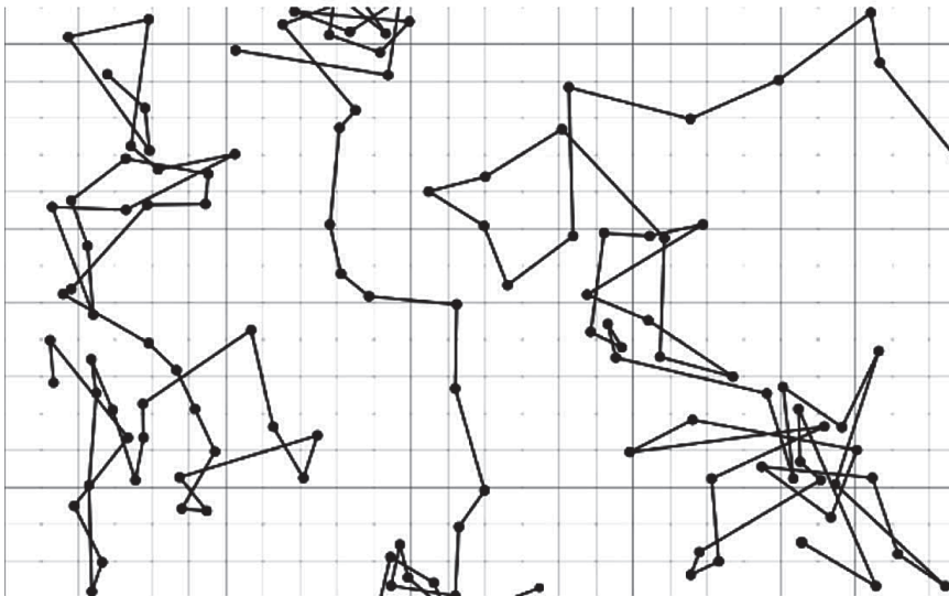
Броунівський рух — шлях часточок пилку у воді під мікроскопом
