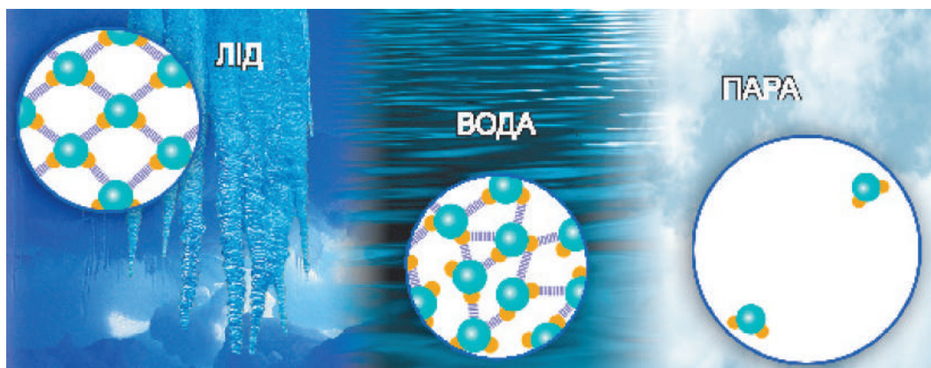
Розташування молекул води у різних її агрегатних станах
