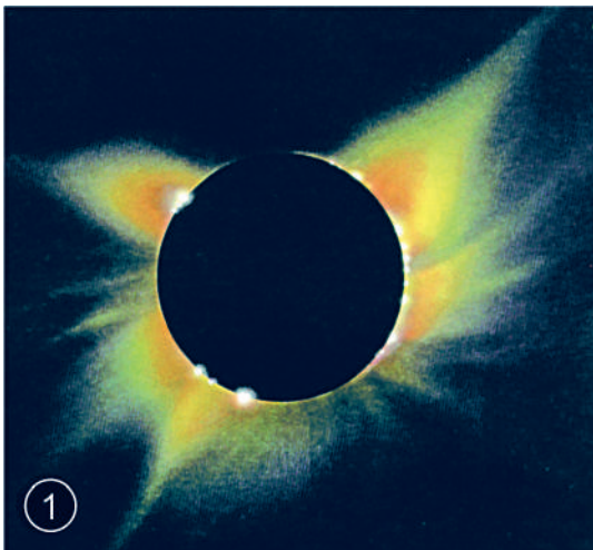
Затемнення Сонця (1) та Місяця (2)
